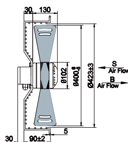
冷却风扇
