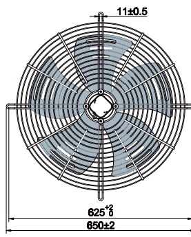
标准风扇
