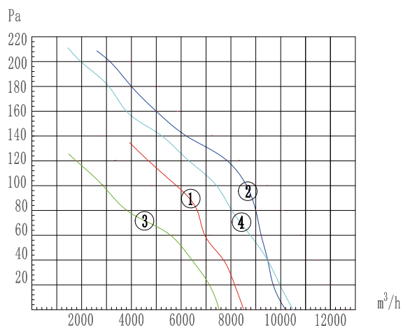
性能曲线
