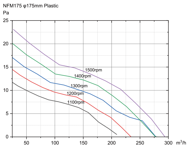
性能曲线
