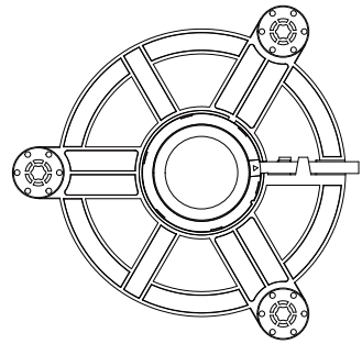
外形尺寸
