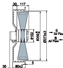
冷却风扇
