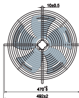
标准风扇
