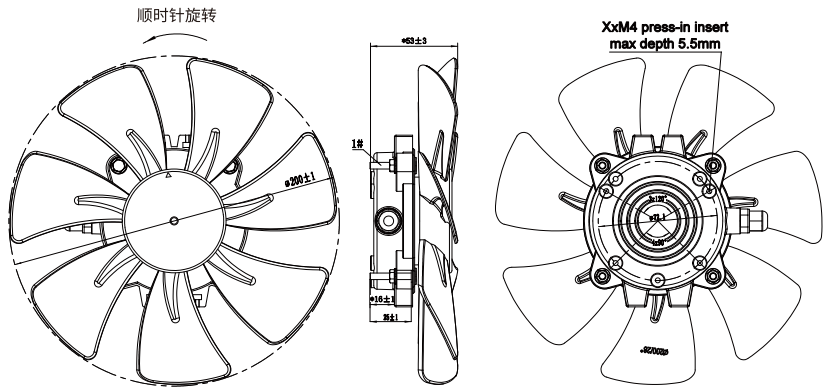
外形尺寸
