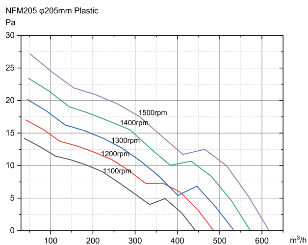
性能曲线
