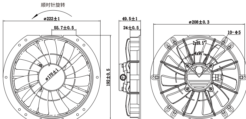
外形尺寸
