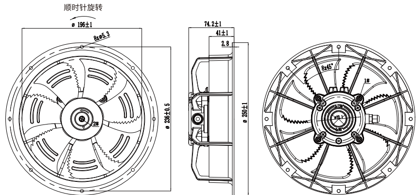
外形尺寸
