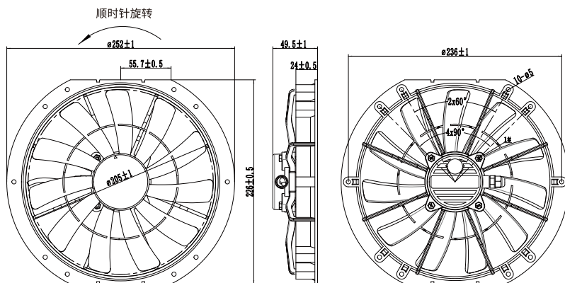
外形尺寸
