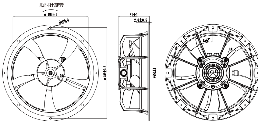
外形尺寸
