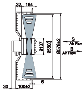
冷却风扇
